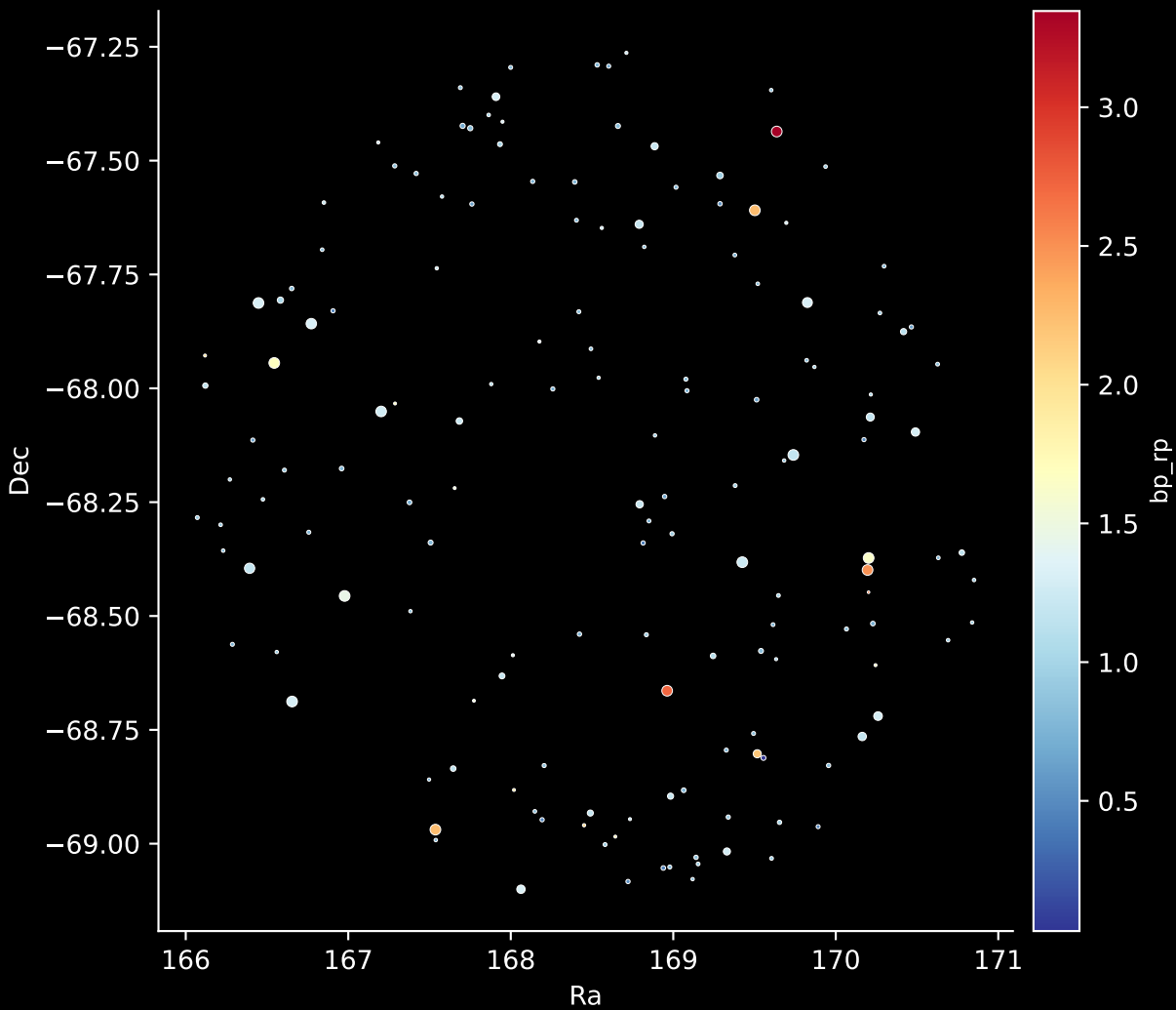
APOGEE DR17 Field: [280-38-O_TESS] Stars: 153
