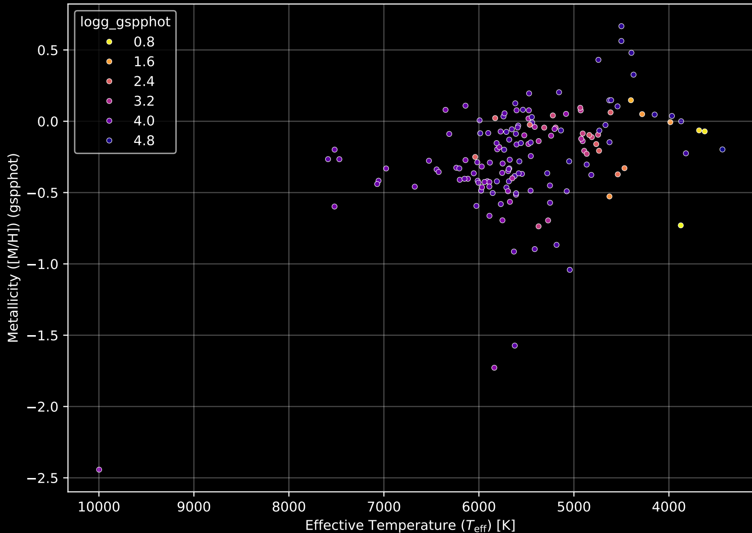
APOGEE DR17 Field: [280-38-O_TESS] Stellar Population Parameters (n= 153)
